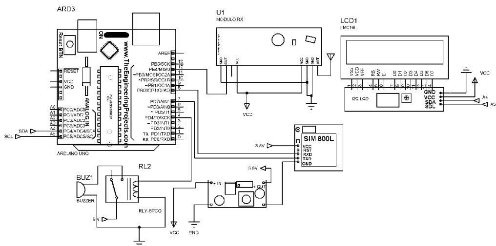
Gambar 6. Rangkaian Skema Reciver Sistem Keamanan Baru
