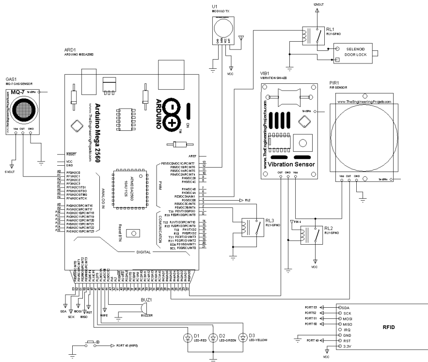
Gambar 5. Rangkaian Skema Transmitter Sistem Keamanan Baru
