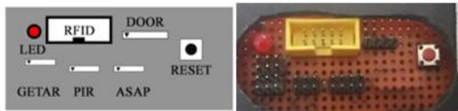
Gambar 8. Implementasi port pada sistem transmitter
