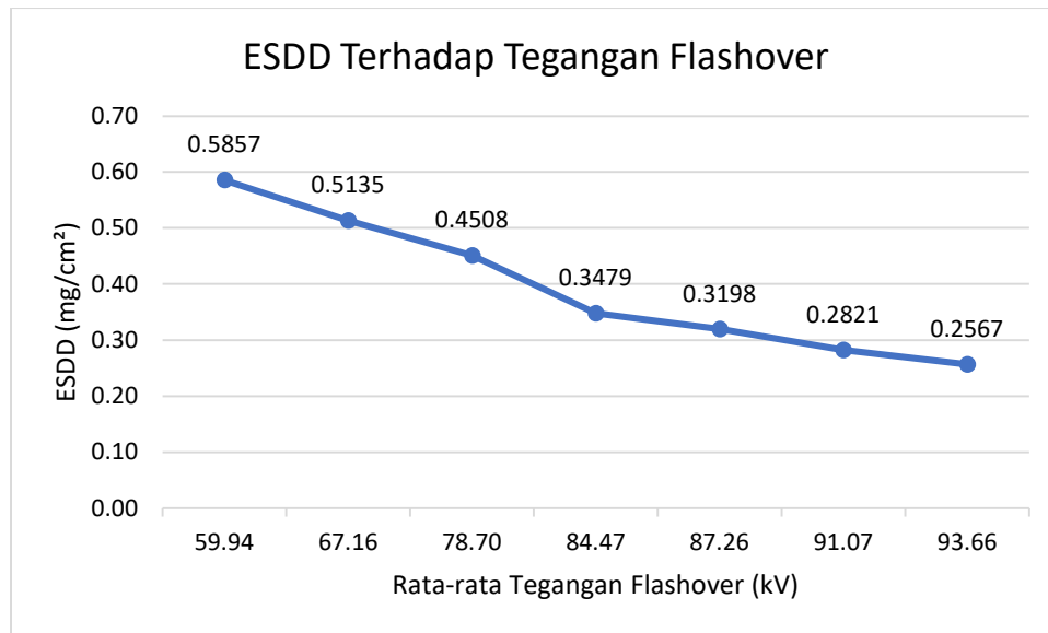
Gambar 4.2 Hubungan ESDD Terhadap Fashover
